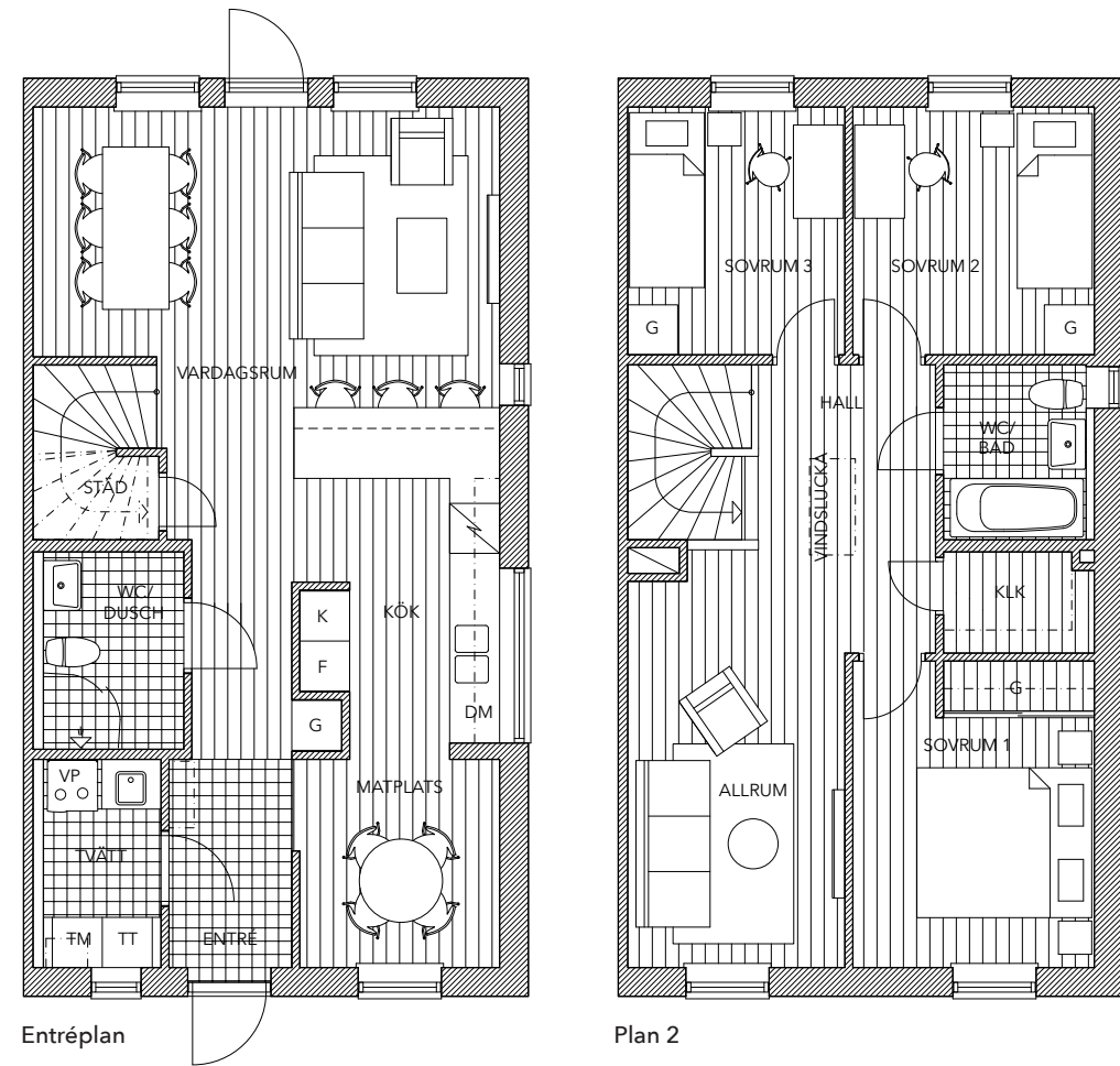
Planlösning hörgavel 5 rok 115 m 2
