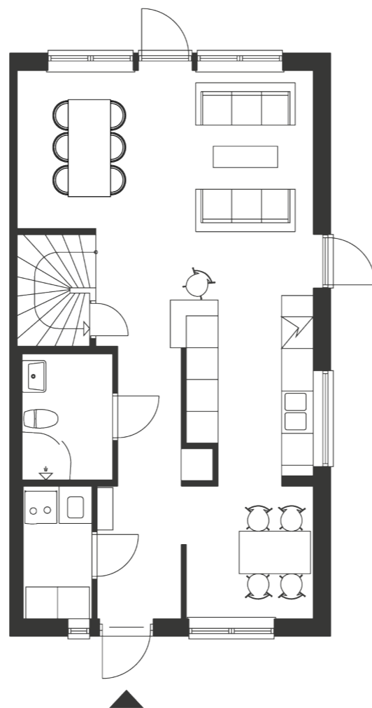
PLAN ETT
