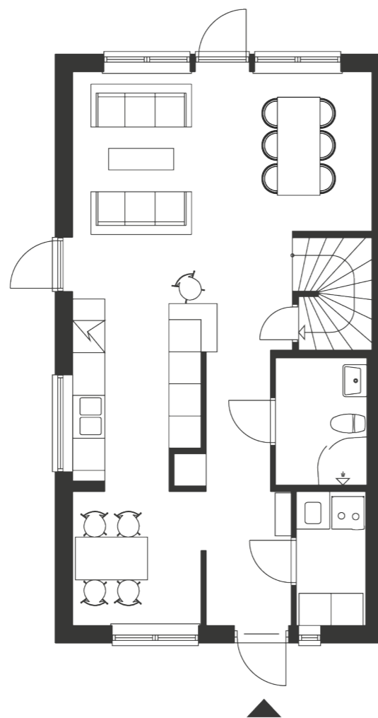
PLAN ETT
