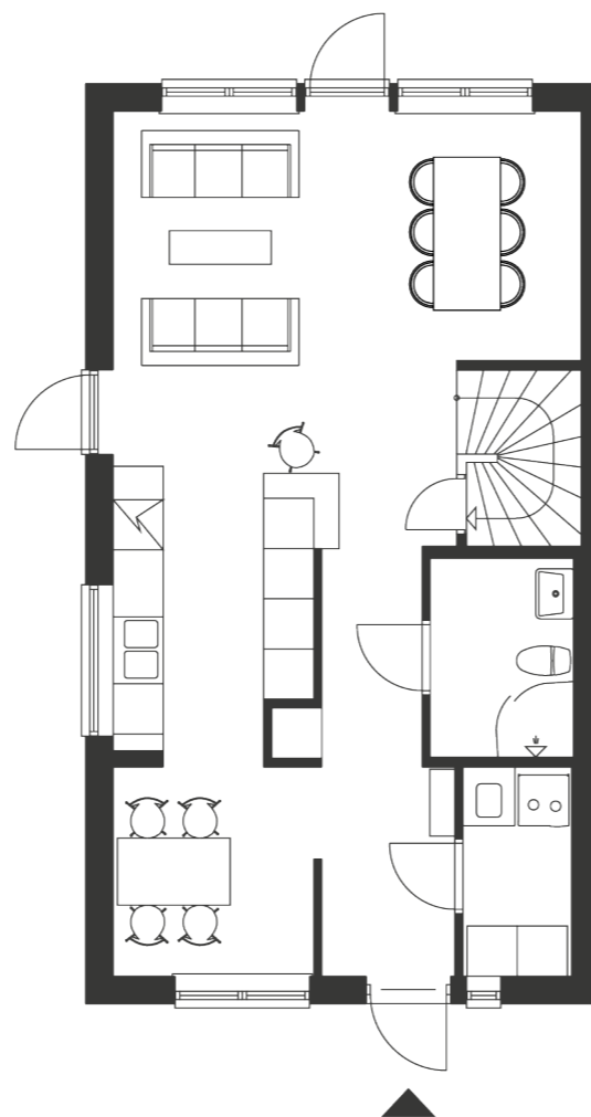
PLAN ETT
